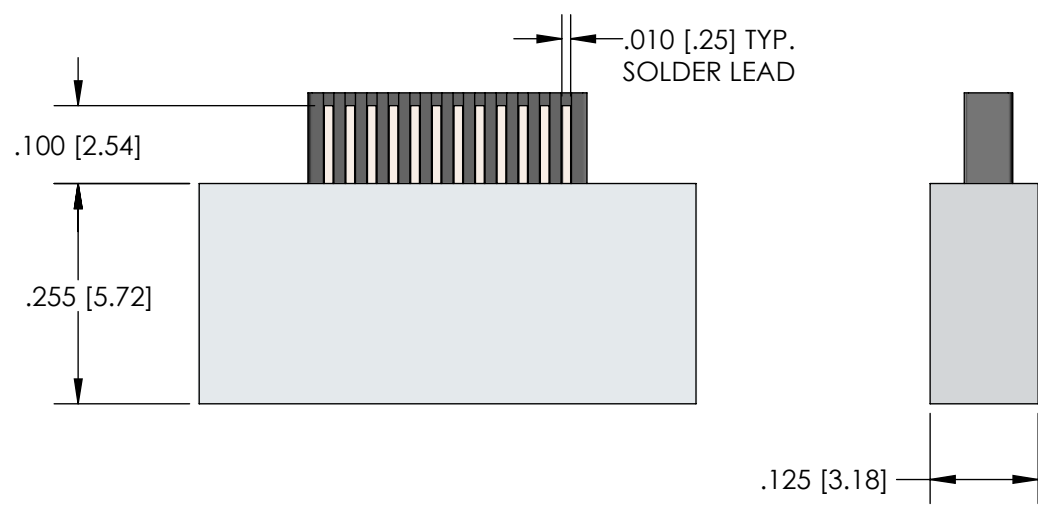
RECEPTACLE (SOCKETS)
