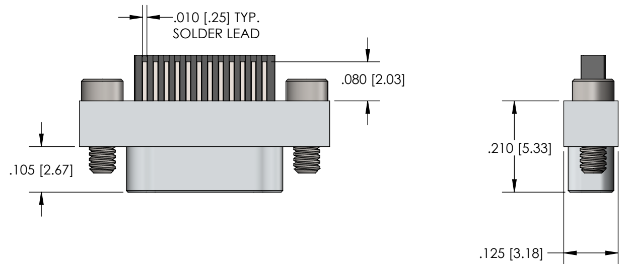
PLUG (PINS)
